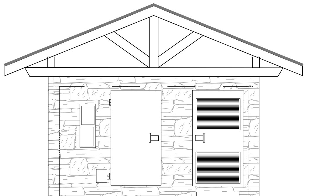
FACADE EST
