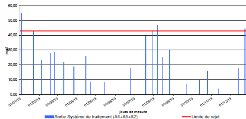
N_NH4 : concentration en sortie du système de traitement les jours de mesures
